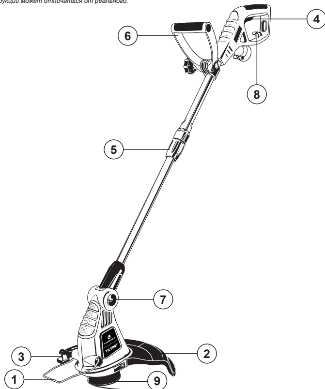
Рис.2. Расположение основных элементов электротриммера:
